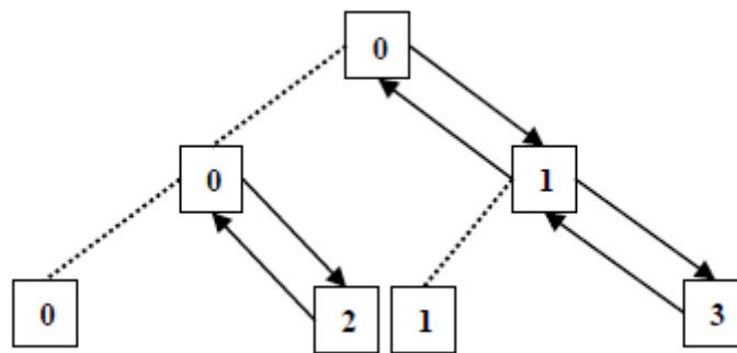
ნახ. 1: MPI-ს პროცესების ხე რეკურსიული merge sort-ისათვის. ისრებით გამოხატულია კომუნიკაცია დამხმარე პროცესებთან, ხოლო წყვეტილი ხაზებით - მონაცემები, რომლებიც რჩება პროცესში შემდგომი სორტირებისთვის.
